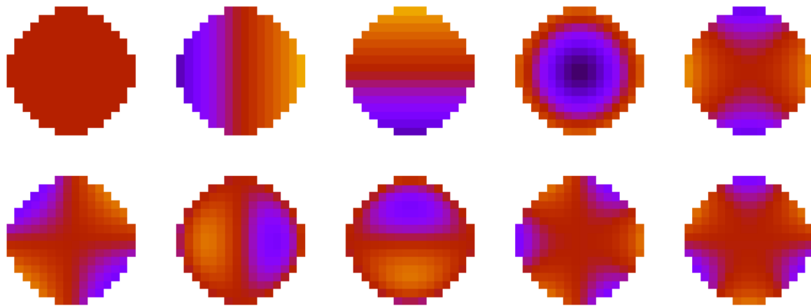
Model波面 (Zernikeモード)
