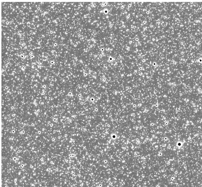
銀河系バルジのRoman field
